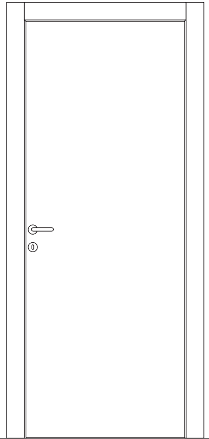
Telaio con coprifilo standard da 100 mm a 130 mm Frame with standard architrave from 100 to 130mm
